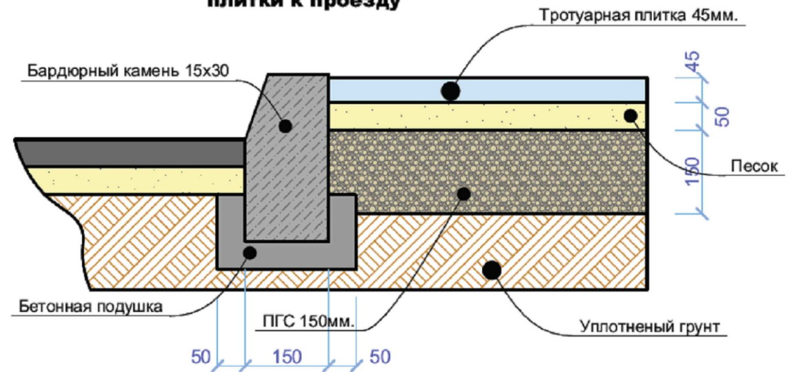
Схема устройства примыкания тротуарной плитки к проезду
