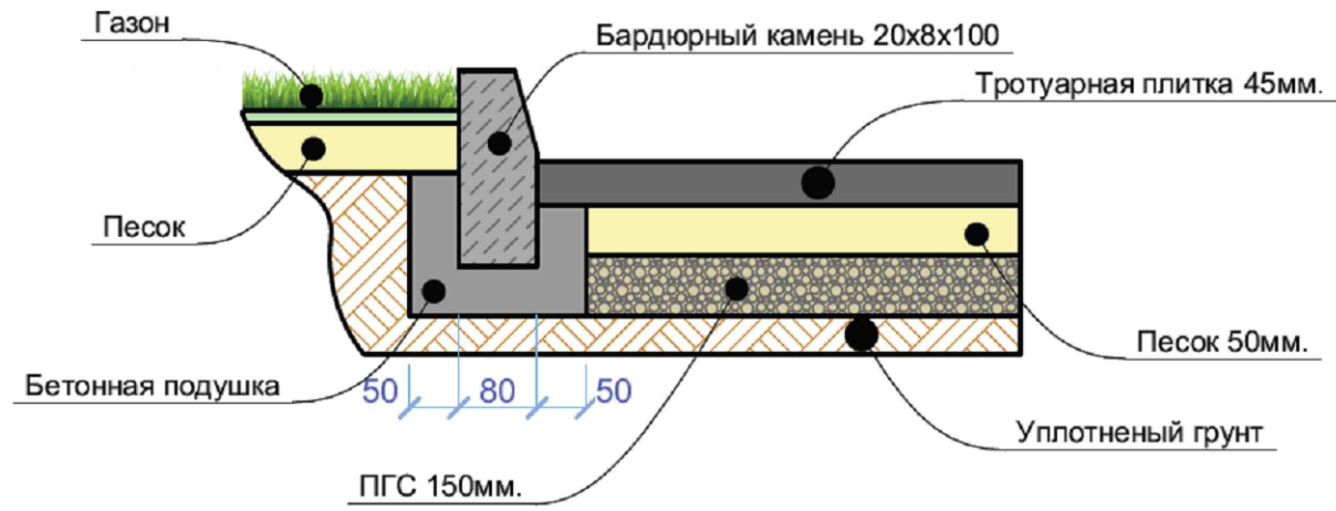
Схема устройства примыкания тротуарной плитки к газону
